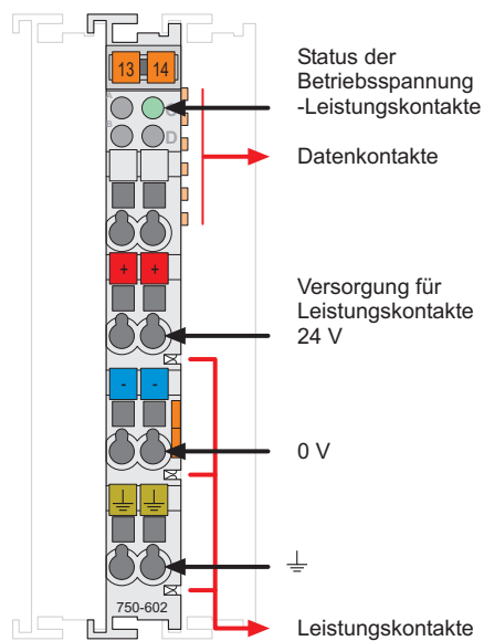
Abb. 2.1.1-1: Potentialeinspeiseklemme 750-602
