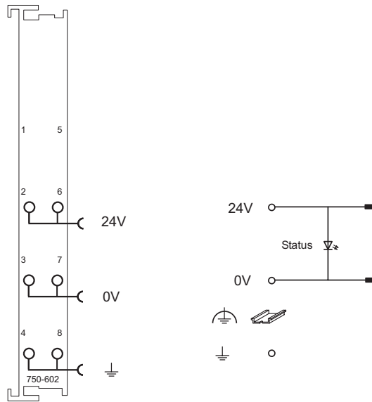
Abb. 2.1.1-3: Potentialeinspeiseklemme 750-602
