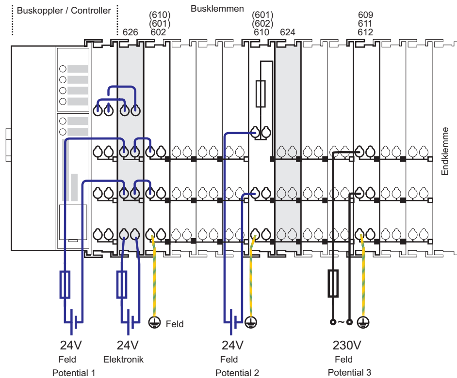
Abb. 2.1.1-4: Einspeisekonzept
